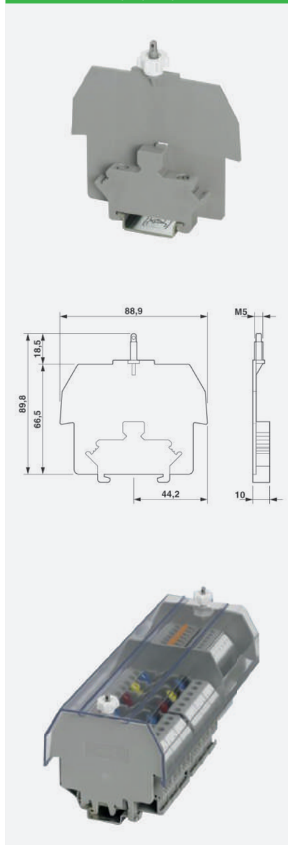
Держатель для защитного профиля со встроенным концевым стопором на монтажную рейку NS 35/7,5
