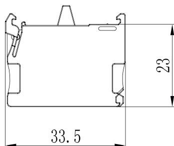
Блок контактов
